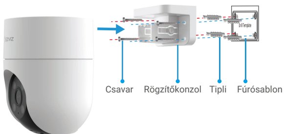
2. ábra Fali rögzítés
