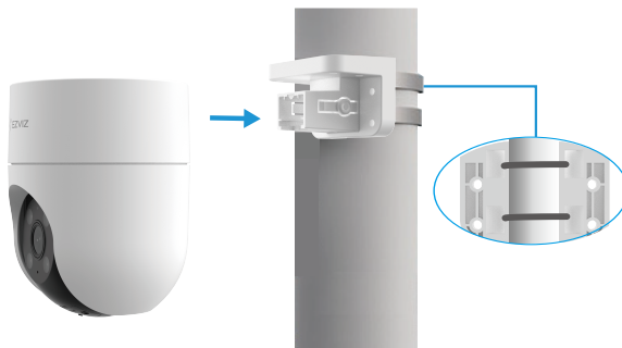
3. ábra Rögzítés oszlopra
