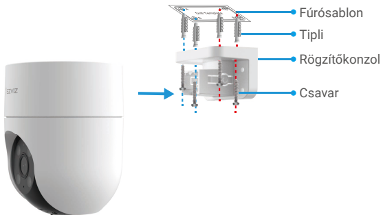
1. ábra Mennyezeti rögzítés
